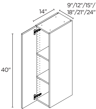
WALL 40" HIGH / 1 DOOR
