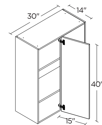
BLIND CORNER WALL 40" HIGH / 1 DOOR
