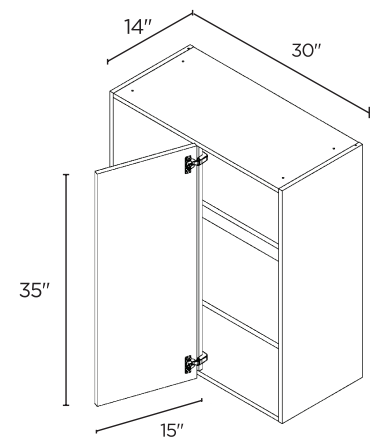
BLIND CORNER WALL 35" HIGH / 1 DOOR
