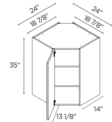
CORNER WALL 35" HIGH / 1 DOOR
